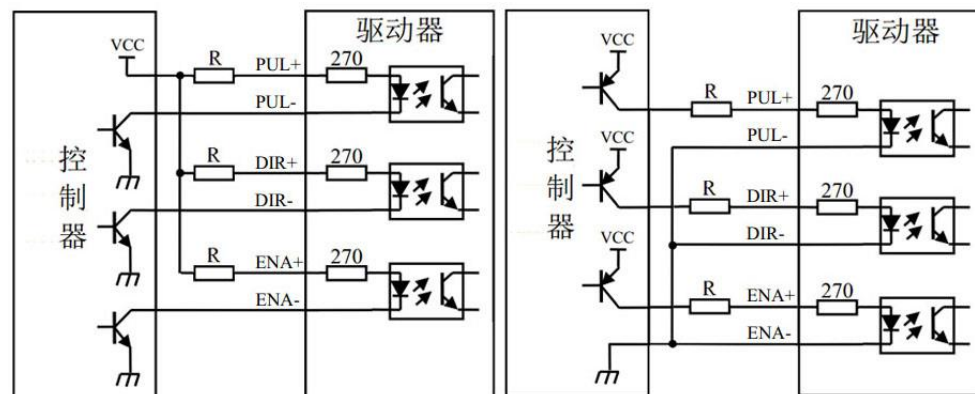
图 2 共阳极接法
