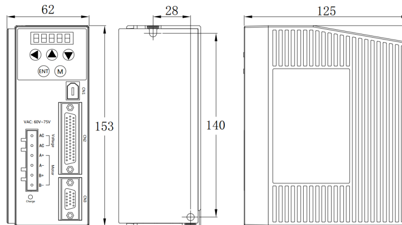
图 1 驱动器安装尺寸图
