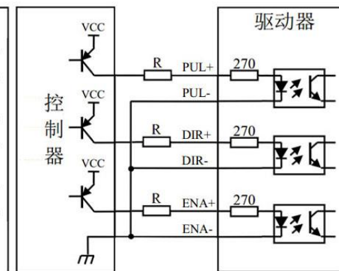
图 3 共阴极接法
